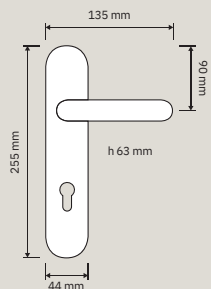
1210 PG 075 Pomolo a girare con rosetta art.075 / Turnable knob on rose art.075
