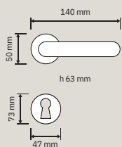
1210 PT 080 Pomolo a tirare / Fixed knob
