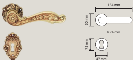
1560 RB 078 Maniglia con rosetta art.078 / Door handle on rose ar t.078
