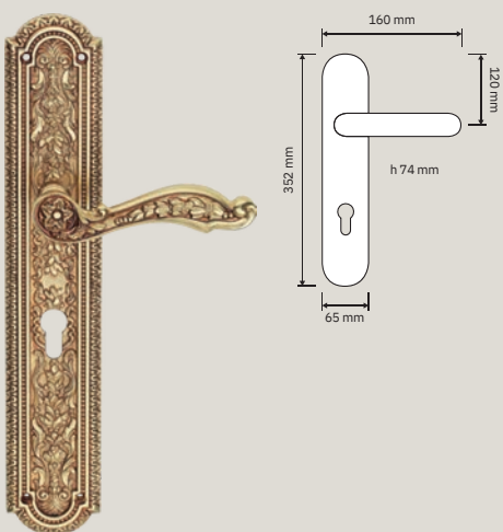
1560 PL Maniglia con placca / Door handle on plate
