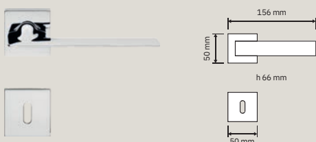
1425 RB 024 Maniglia con rosetta art.024 / Door handle on rose ar t.024
