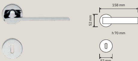
1425 RB 023 Maniglia con rosetta art.023 / Door handle on rose ar t.023
