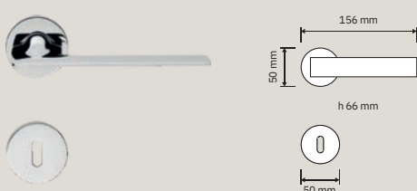
1425 RB 025 Maniglia con rosetta art.025 / Door handle on rose ar t.025
