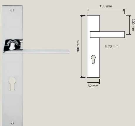
1425 PL Maniglia con placca / Door handle on plate
