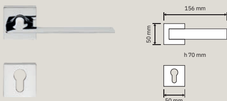
1425 RB 019 Maniglia con rosetta art.019 / Door handle on rose art.019
