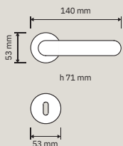
1395 SL Maniglione su placca / Pull handle on plate
