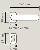
1395 DK Maniglia per finestra con movimento DK 4 posizioni / Window handle with DK movement 4 clicks
