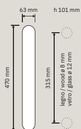
1408 MN 723 Maniglione Crystal. Attenzione: l'interasse può variare leggermente, chiedere sempre le misure prima di forare la porta. / Crystal pull handle. Attention: the distance can have little changes, please always ask before making the holes in the door.
