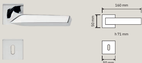
1420 RB 024 Maniglia con rosetta art.024 / Door handle on rose art.024
