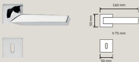
1420 RB 019 Maniglia con rosetta art.019 / Door handle on rose art.019
