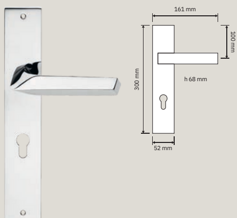
1420 PL Maniglia con placca art.1104 / Door handle on plate art.1104
